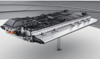
eVito Tourer
